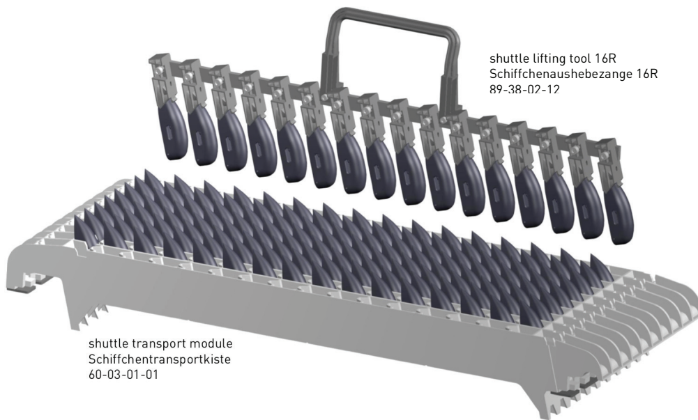
The shuttle transport module is filled with loaded shuttles. Die Schiffli transportkiste wird mit vollen Schiffli bestückt.
